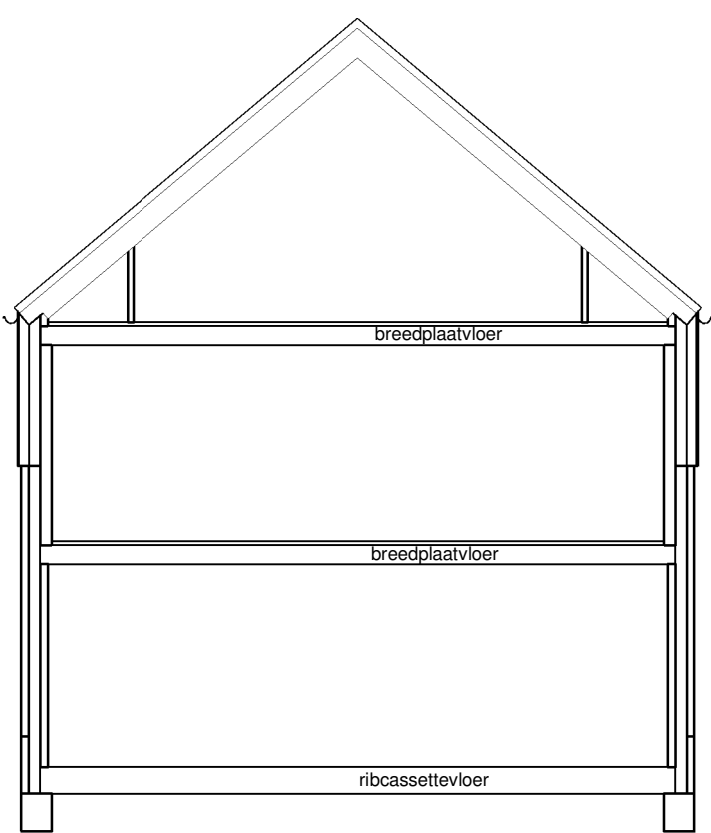
doorsnede 1 : 100
