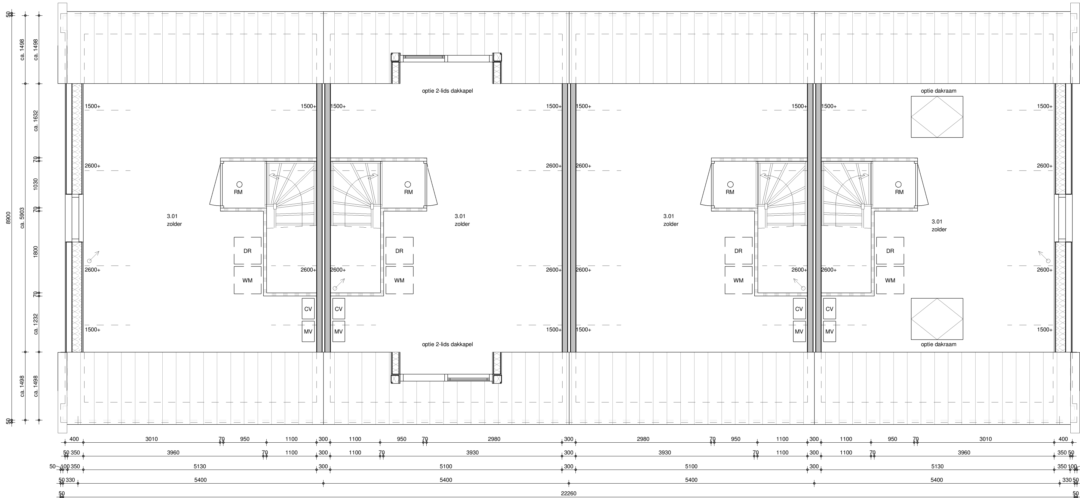
tweede verdieping 1 : 50
