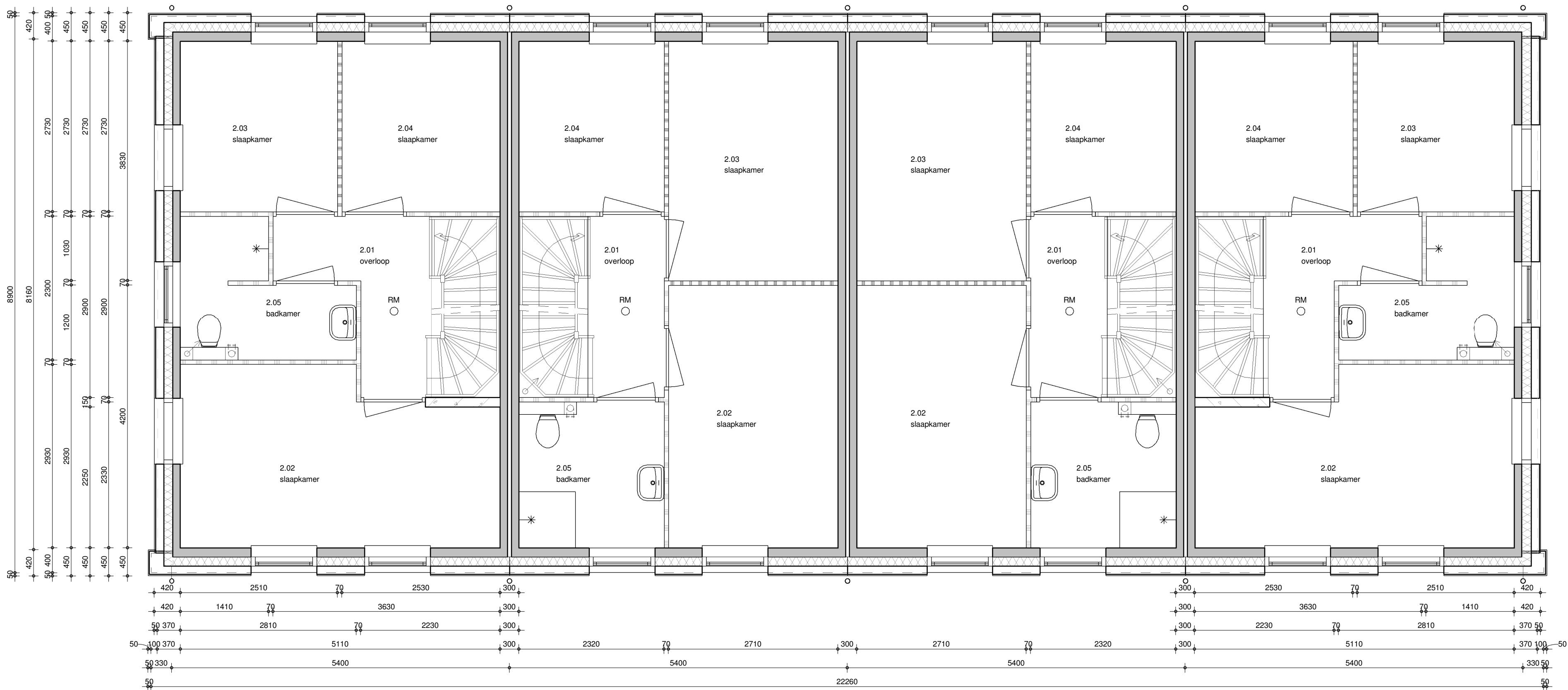
eerste verdieping 1 : 50
