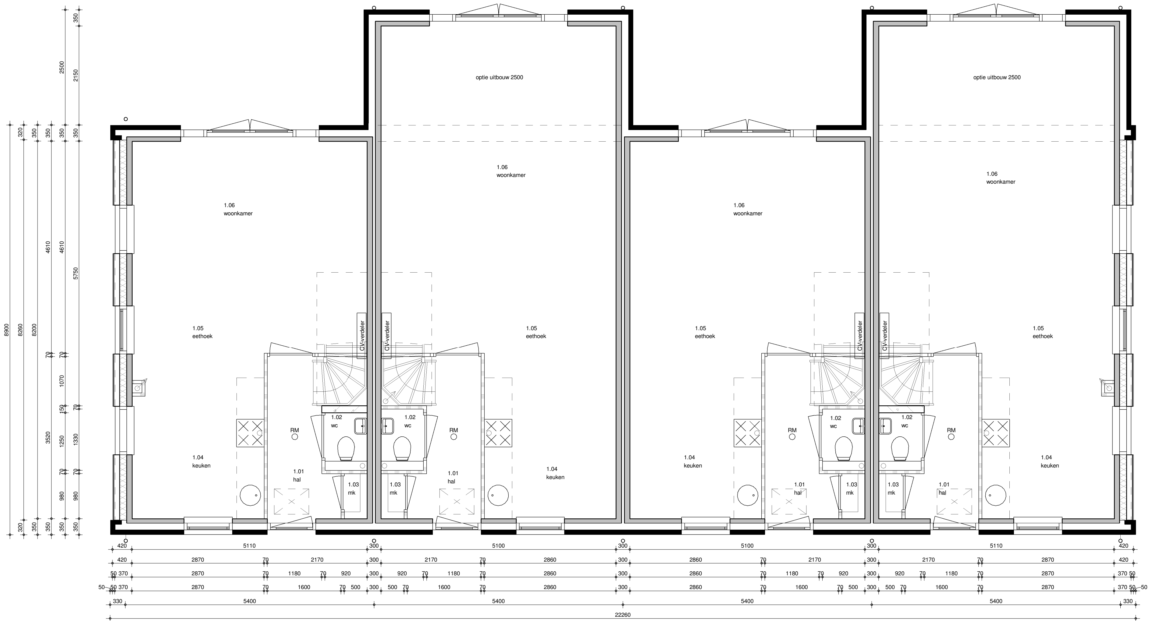
begane grond 1 : 50
