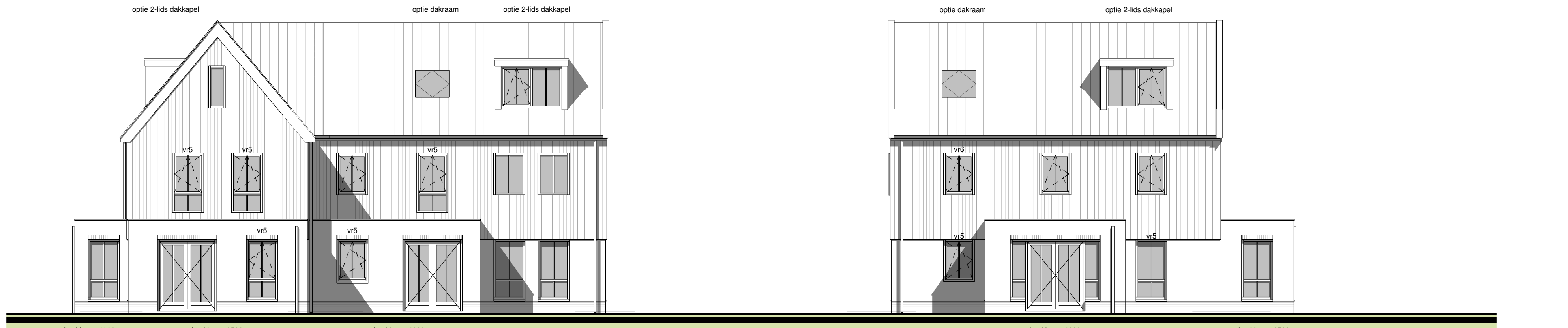
achtergevel 1 : 100
