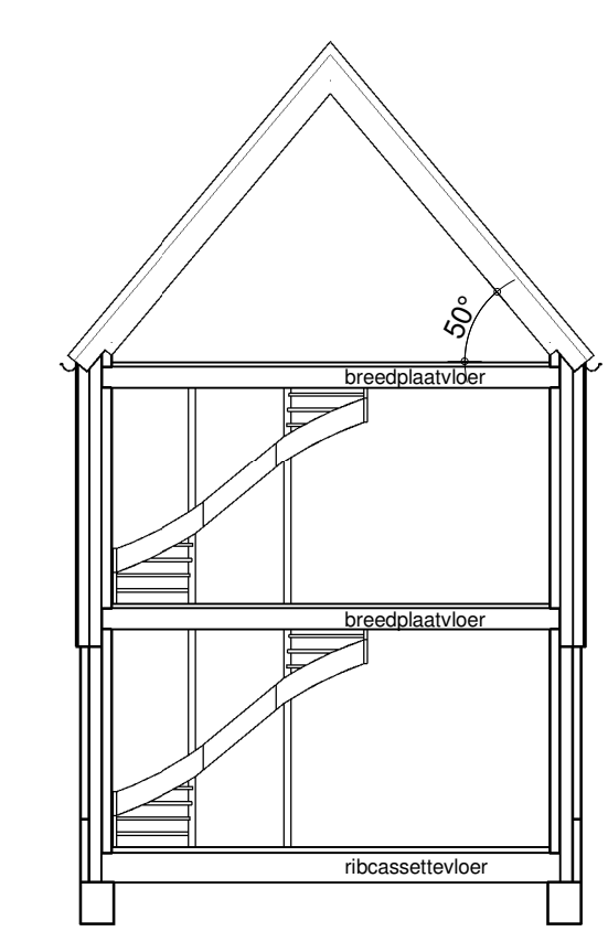
doorsnede A - A 1 : 100
