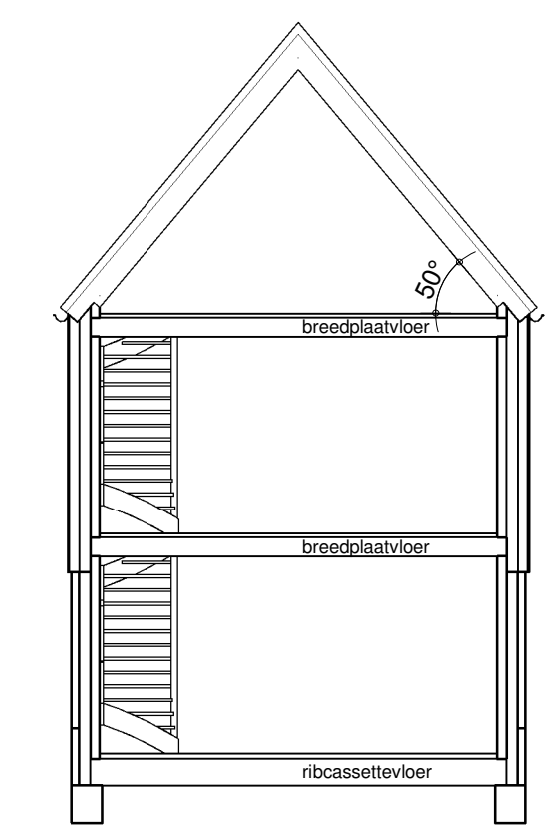
doorsnede B - B 1 : 100
