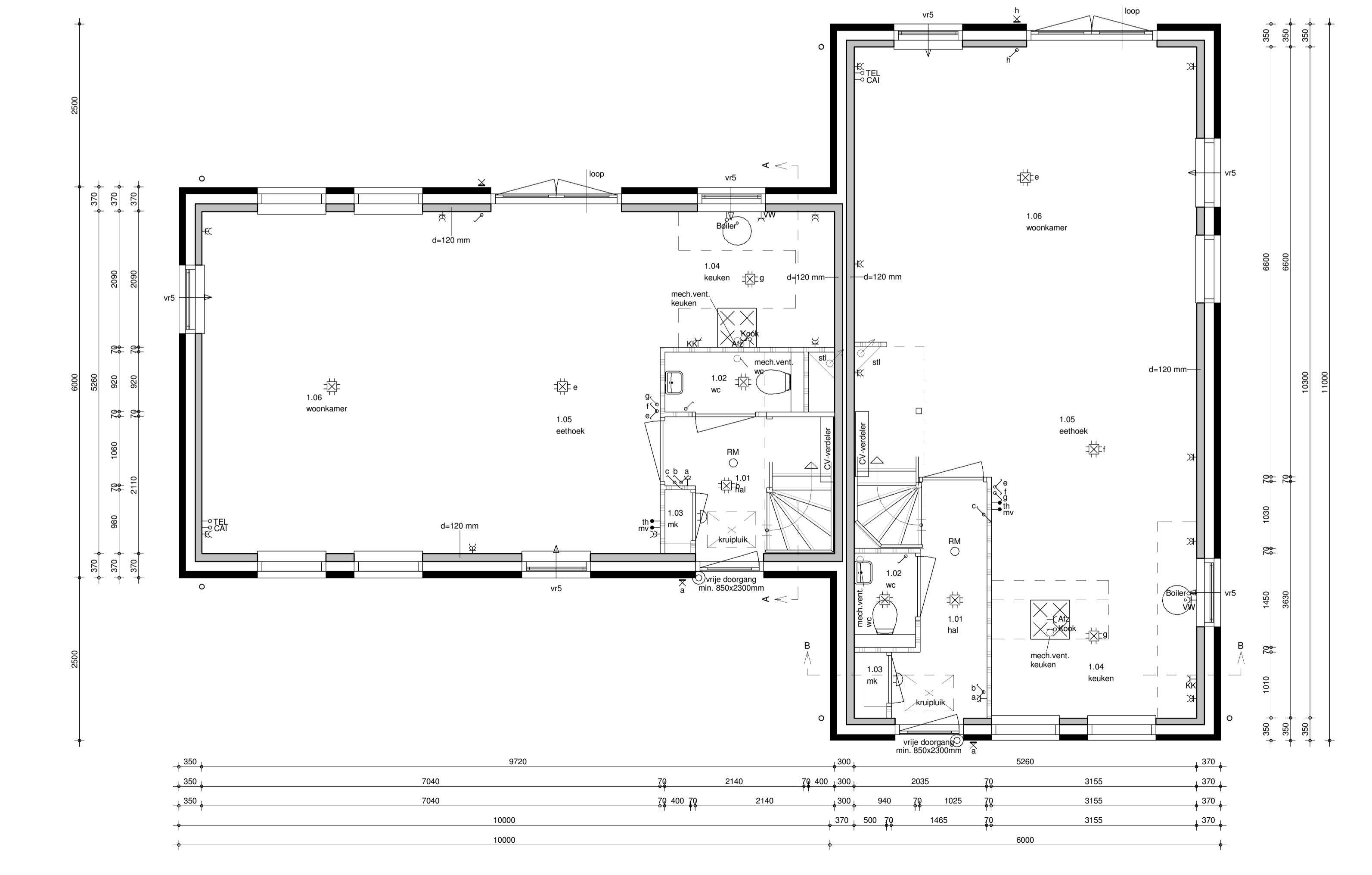
begane grond 1 : 50
