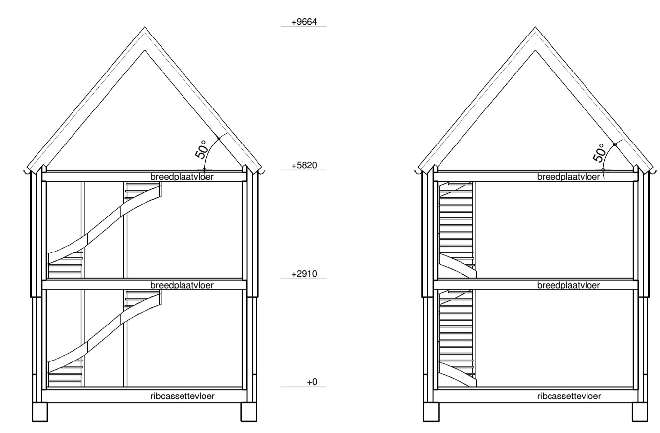
doorsnede A - A 1 : 100
