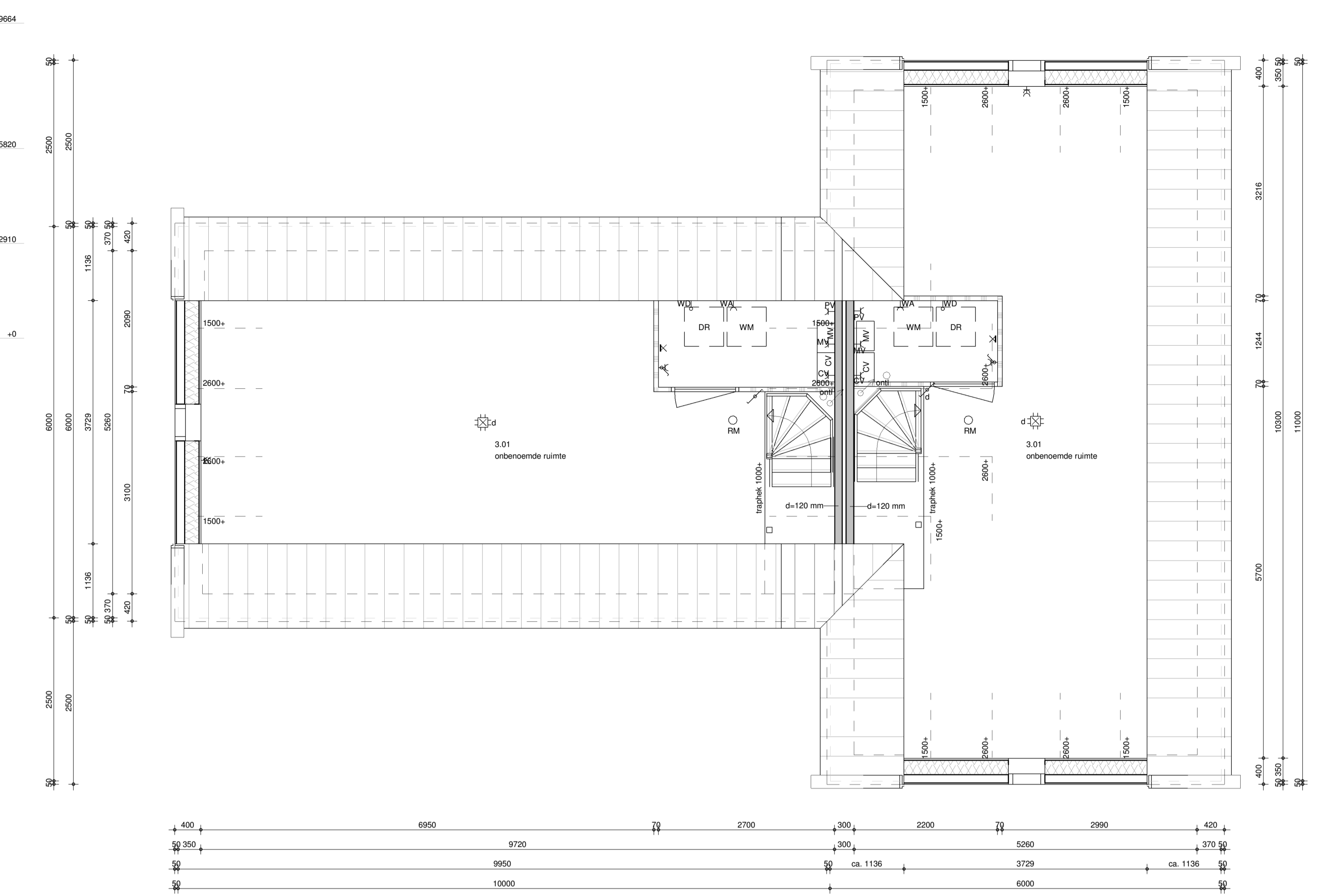
tweede verdieping 1 : 50
