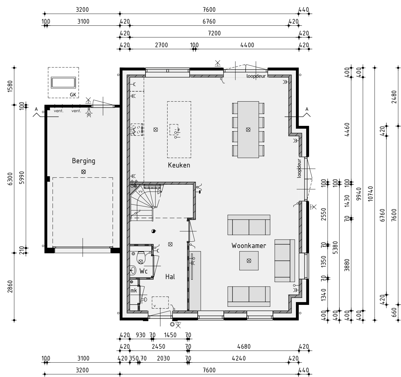
Begane grond
