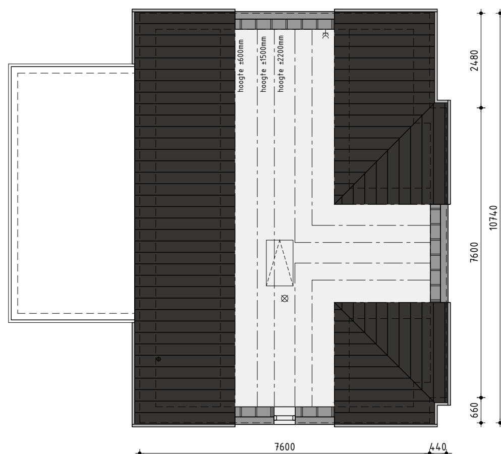
2de Verdieping
