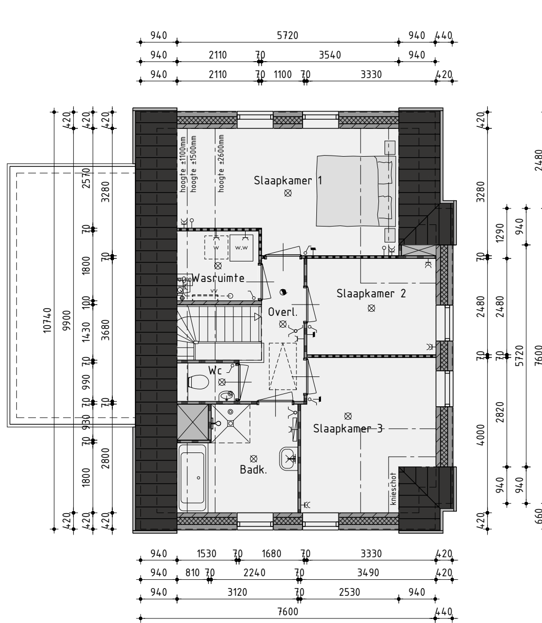
1ste Verdieping
