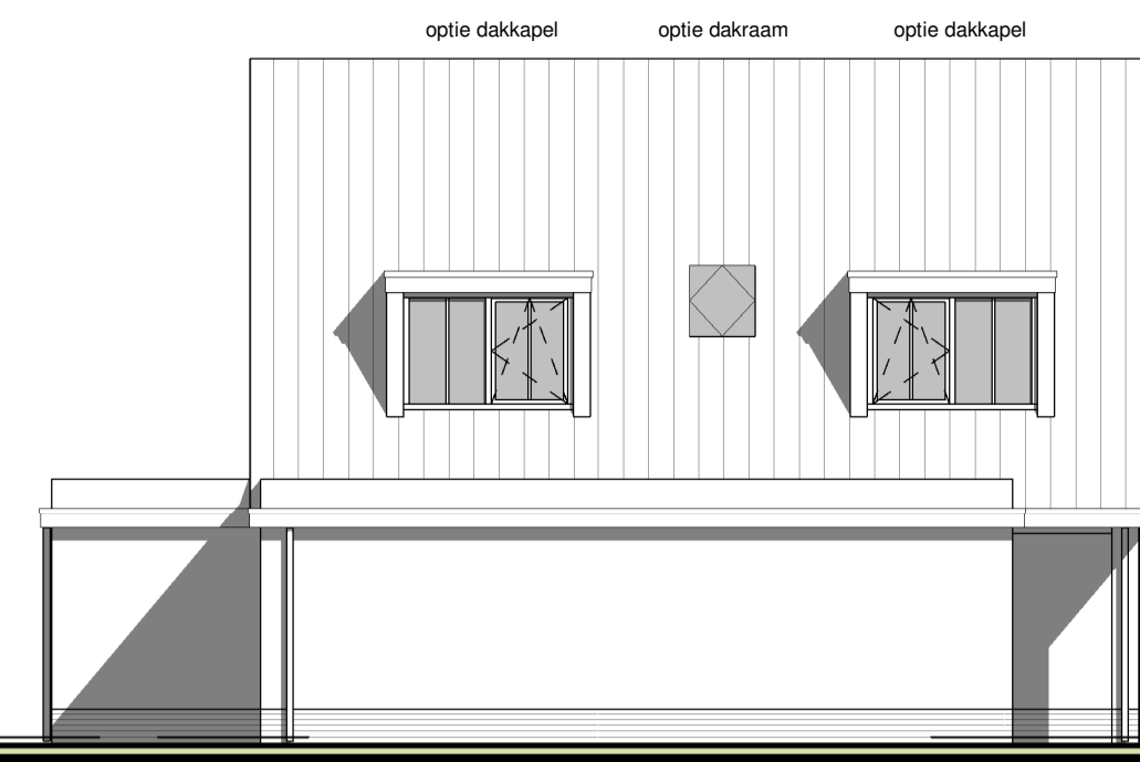
linkergevel 1 : 100
