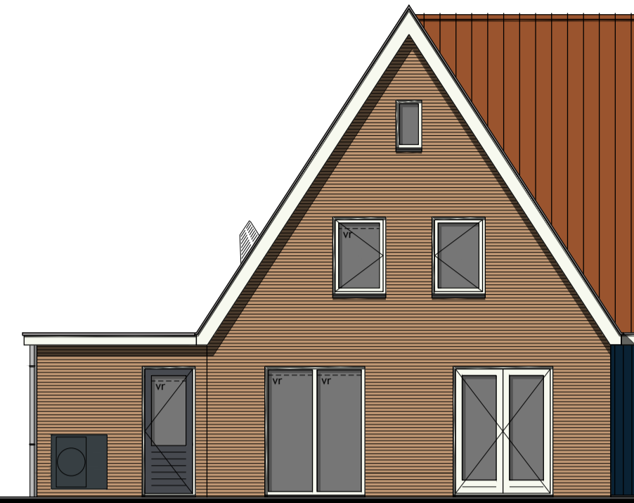
Achtergevel
