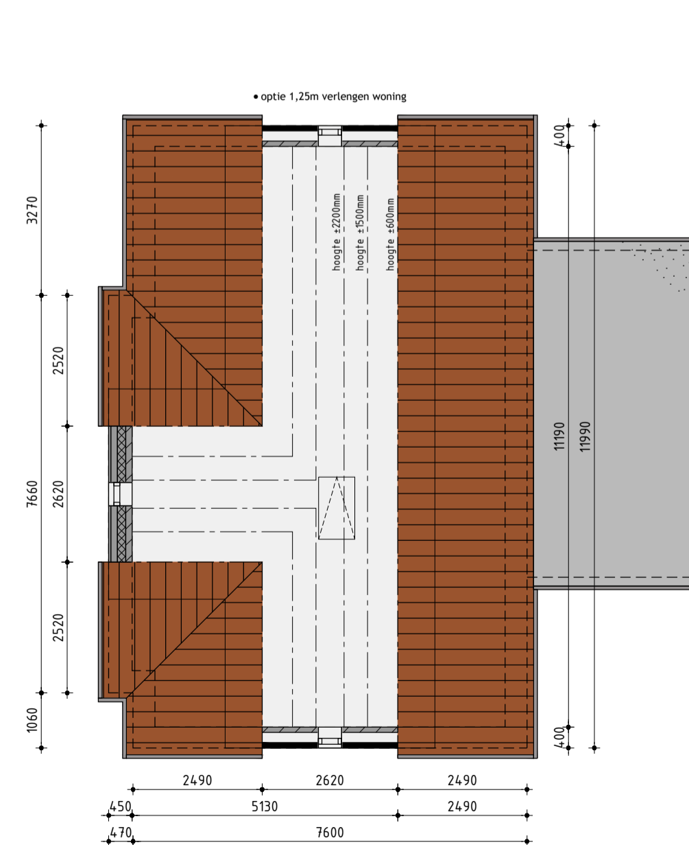
2de Verdieping
