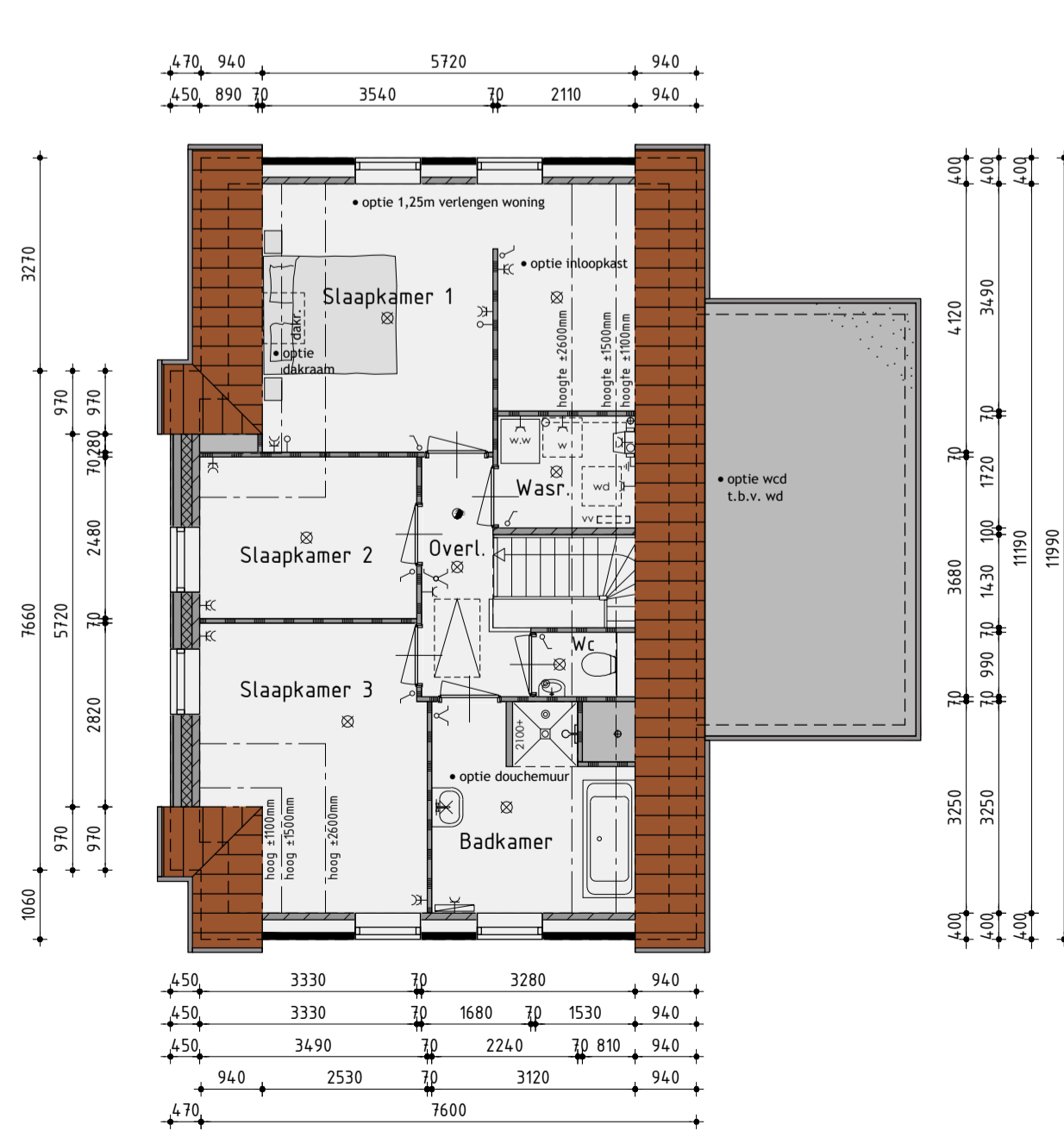
1ste Verdieping
